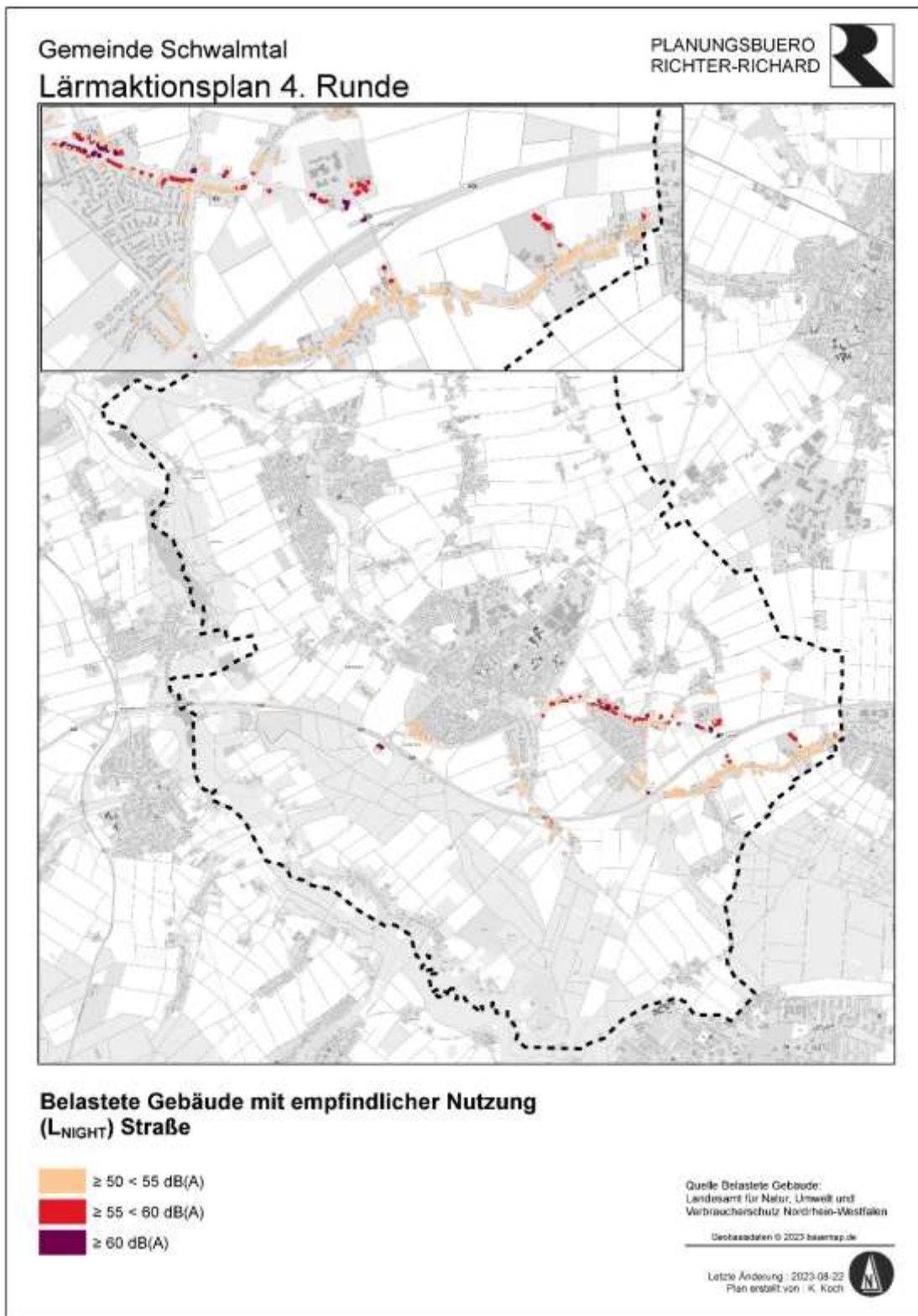
Abb. 5.8: Belastete Gebäude Straßenverkehr L_{night} \geq 50 \text{ dB(A)}
